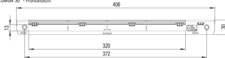
ZUMGN 30° - Frontansicht
