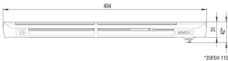
ZUOGN 30° - Frontansicht
